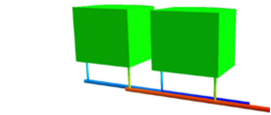
1차원 유동 해석 기능을 활용한 탱크 - 파이프 연계 시스템 해석
