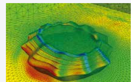
압력분포
