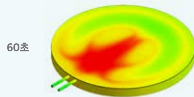
전위차로 인한 웨이퍼 척의 가열
