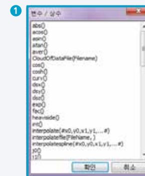
함수 선택
