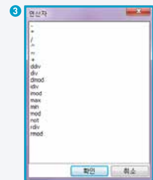
기본 연산자
